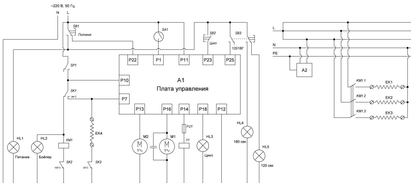
Рисунок 7 Схема электрическая принципиальная Silanos E-50PS
